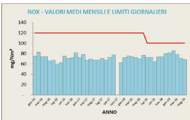
Grafici 27 e 27a: Valori medi e limiti per impianto a pieno regime di NH3 e NOX
