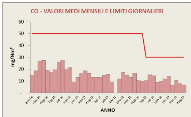
Grafici 26 e 26a: Valori medi e limiti per impianto a pieno regime di CO e COT
