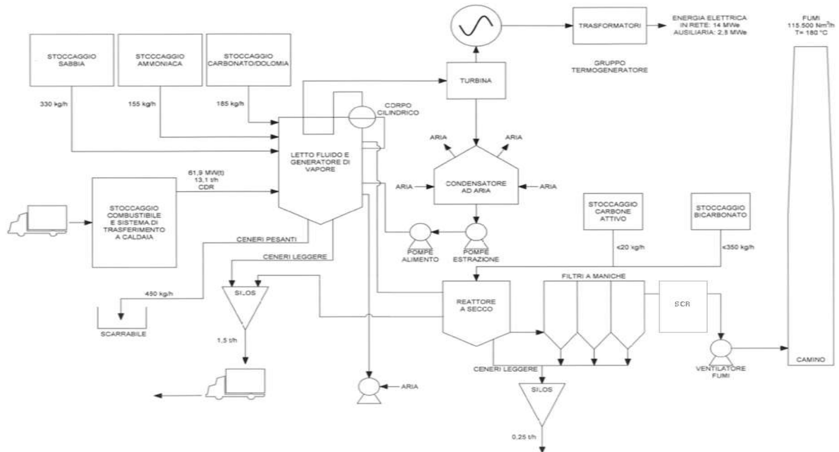
Fig. n. 5 – Layout Centrale
