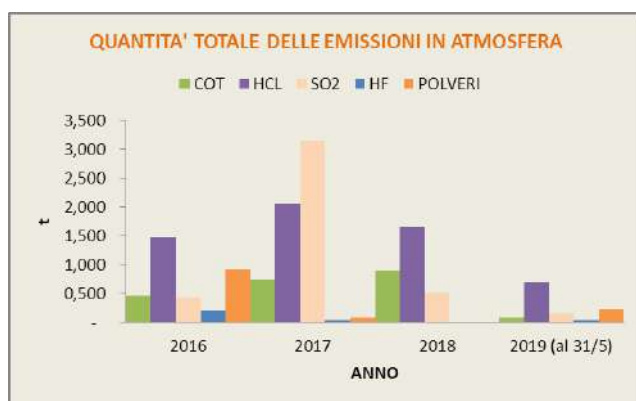
Grafici 22 e 22a: Quantità di inquinanti emessi su base annuale.
