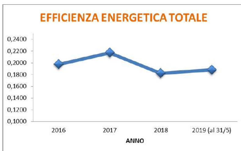
Grafico 4: Efficienza energetica
