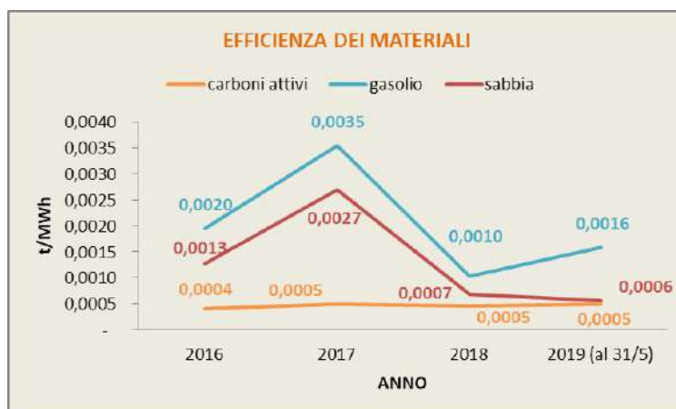
Grafico 14: Efficienza carboni attivi, calcare dolomite e sabbia
