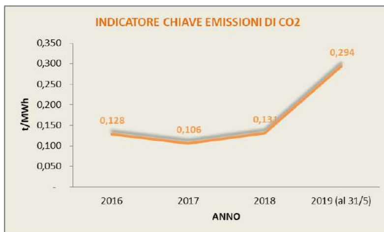
Grafico 25: Rapporto fra CO2 emessa in atmosfera ed EEPL
