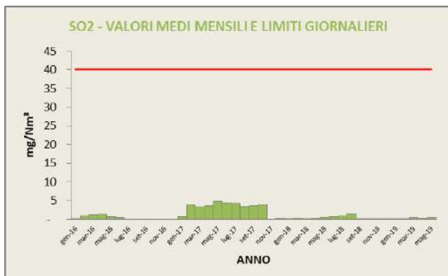
Grafici 28 e 28a: Valori medi e limiti per impianto a pieno regime di SO 2 e HF
