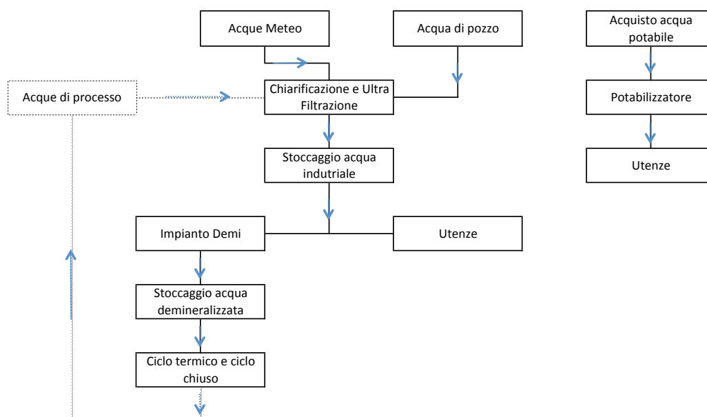
Fig. n. 29 – Schema di flusso delle acque
