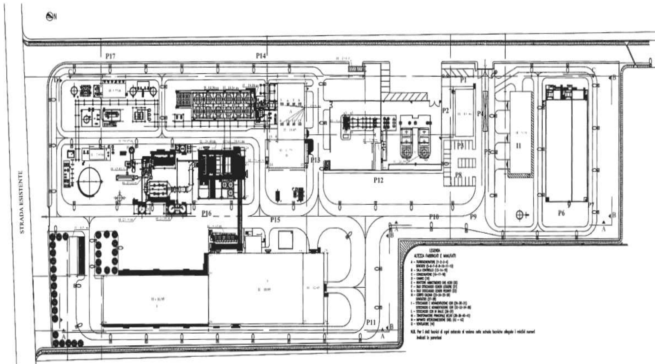
Fig. 40 Planimetria intero stabilimento, con punti di misura dei campi elettromagnetici
