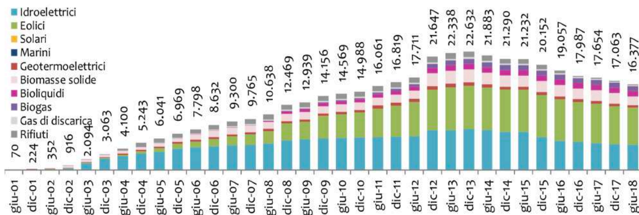
Fig. 41 Evoluzione storica degli impianti che hanno ottenuto la qualifica IAFR dal GSE in Italia (Fonte GSE)
