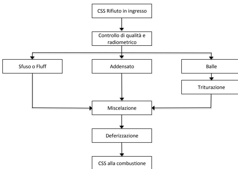
Fig. n. 6 – Diagramma di flusso di preparazione del combustibile
