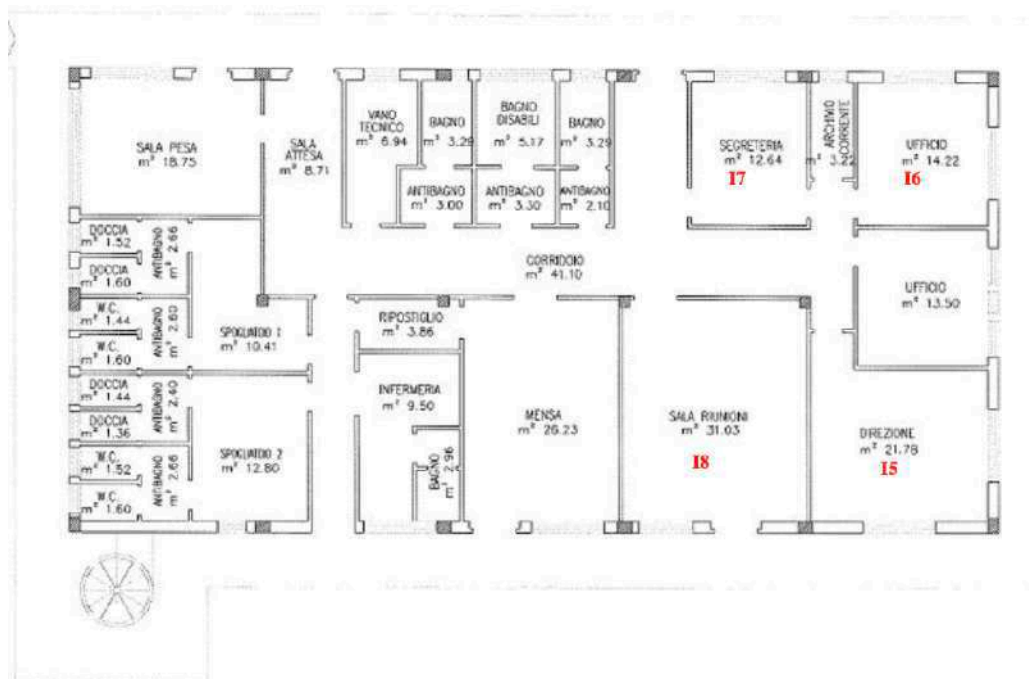
Fig. 10 Planimetria intera fabbricato turbogeneratore e palazzina uffici, con punti di misura dei campi elettromagnetici
