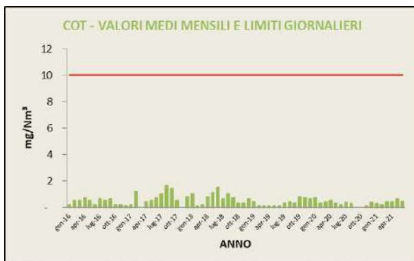
Grafici 27 e 27a: Valori medi e limiti per impianto a pieno regime di CO e COT
