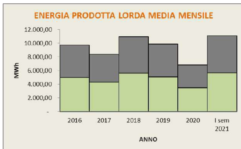
Grafico 1: Energia elettrica prodotta lorda media mensile e quota rinnovabile
