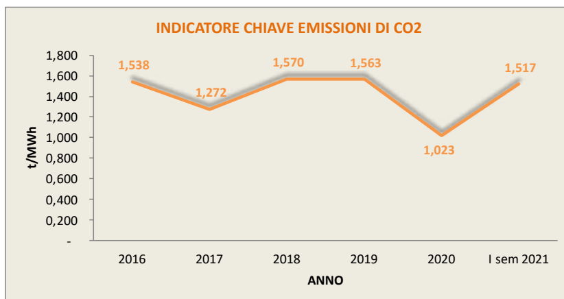
Grafico 25: Rapporto fra CO2 emessa in atmosfera ed EEPL
