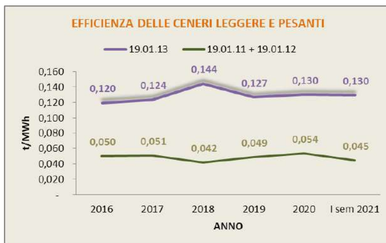
Grafico 20: Efficienza di ceneri leggere e pesanti apprezzabile visivamente
