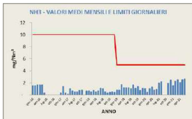
Grafici 28 e 28a: Valori medi e limiti per impianto a pieno regime di NH3 e NOx
