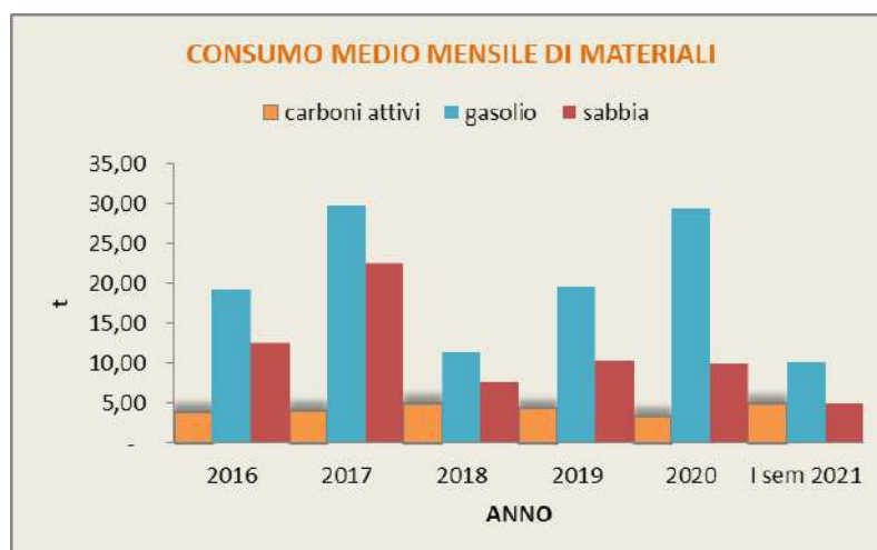
Grafico 11: Consumo carboni attivi, calcare dolomite e sabbia
