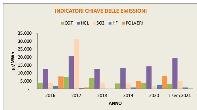
Grafici 24 e 24a: Rapporto fra quantità di inquinanti emesse e EEPL
