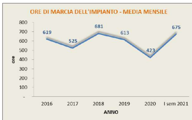
Grafico 6: Ore di marcia dell'impianto media mensile
