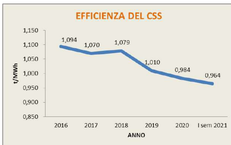
Grafico 12: Efficienza del CSS
