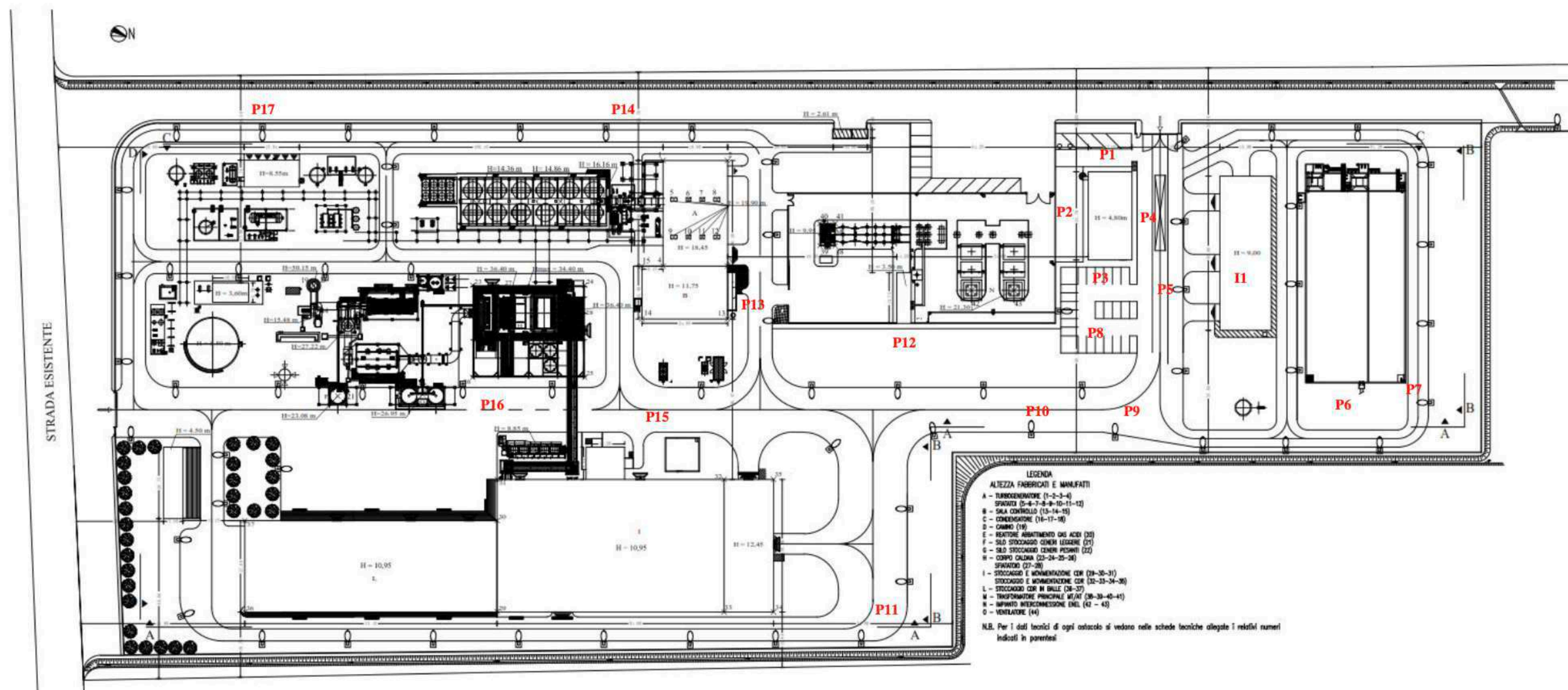
Fig. 9 Planimetria intero stabilimento, con punti di misura dei campi elettromagnetici
