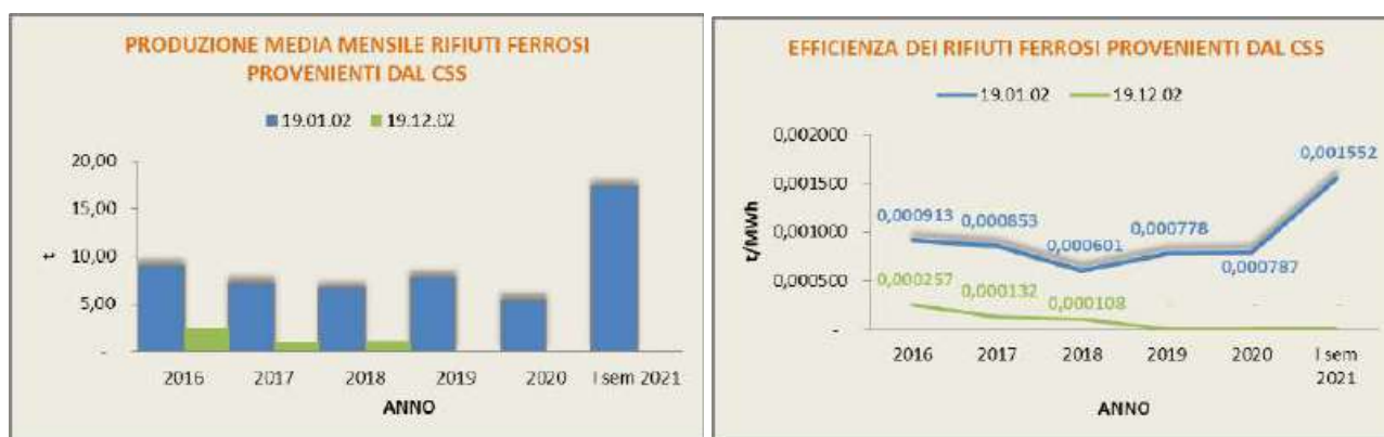
Grafico 18 e 18a: Produzione e efficienza CER 19.01.02 e 19.12.02.
