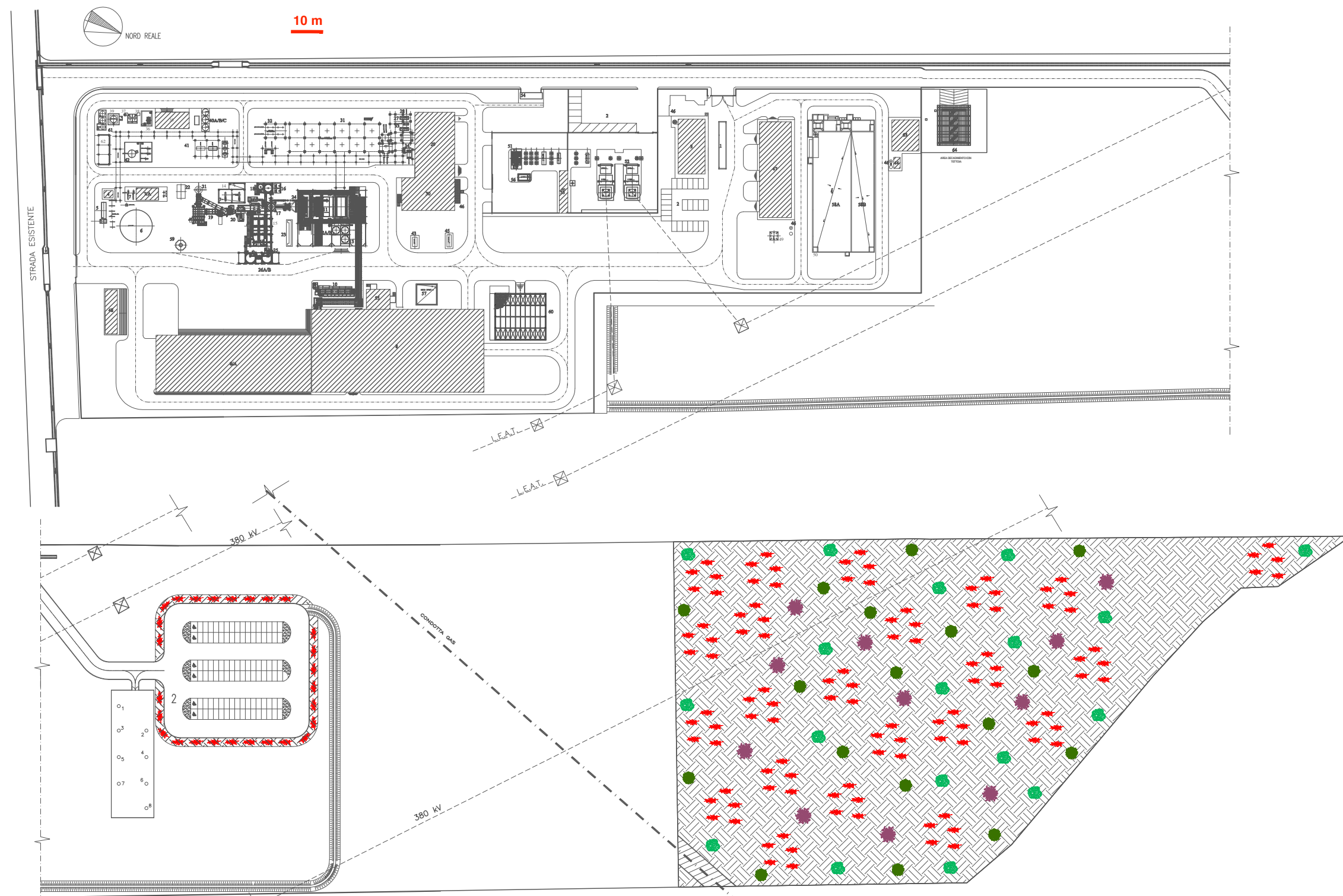
Fig. n. 4 - Planimetria Impianto di Produzione di Energia Elettrica – E.T.A. S.r.l.
