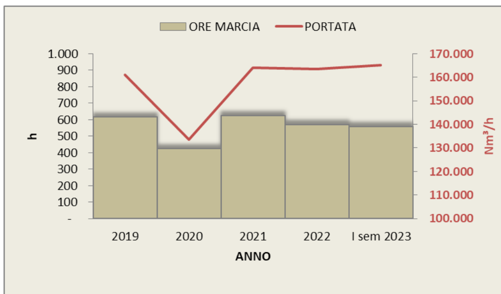
Grafico 23: Ore di marcia e portata su base annuale
