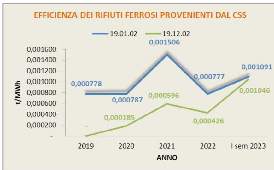
Grafico 18a: Efficienza CER 19.01.02 e 19.12.02.
