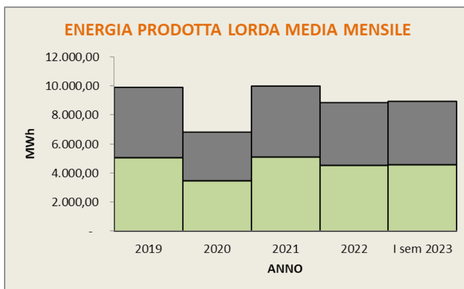
Grafico 1: Energia elettrica prodotta lorda media mensile e quota rinnovabile
