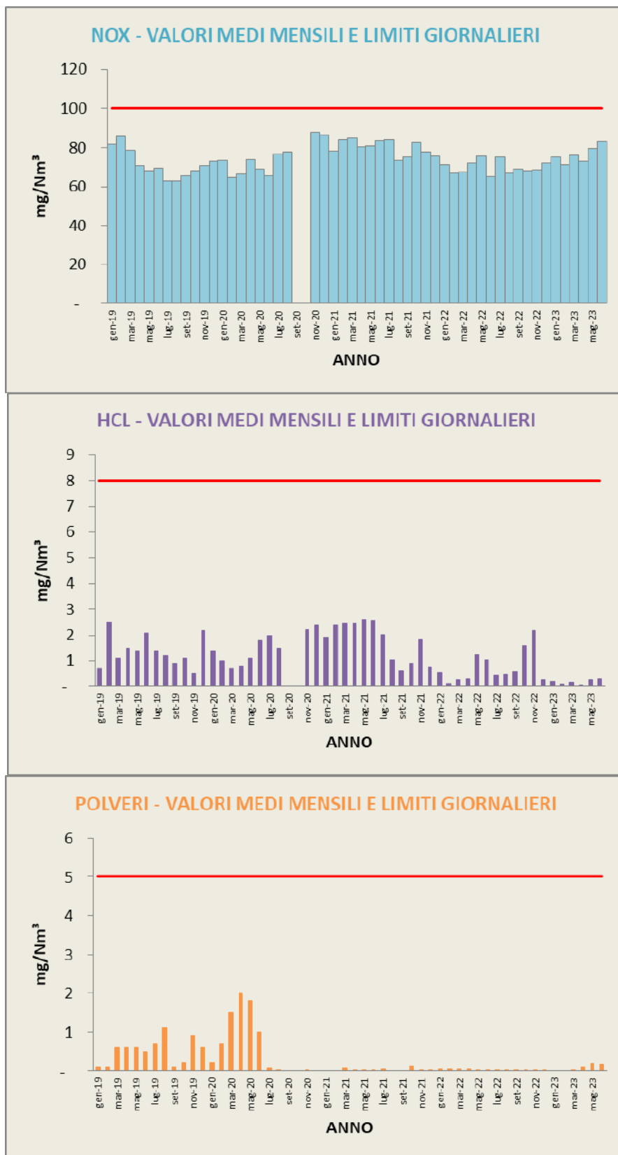
Grafici 28, 28a e 28b: Valori medi e limiti per impianto a pieno regime di NO x , HCl e Polveri.
