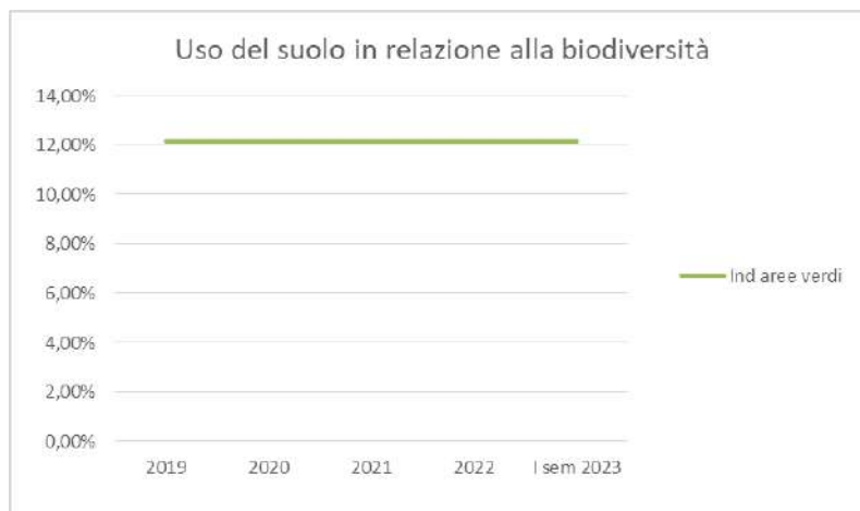
Grafico 21: Indice di Biodiversità risultato dal rapporto fra sup. edificata e sup. disponibile.
