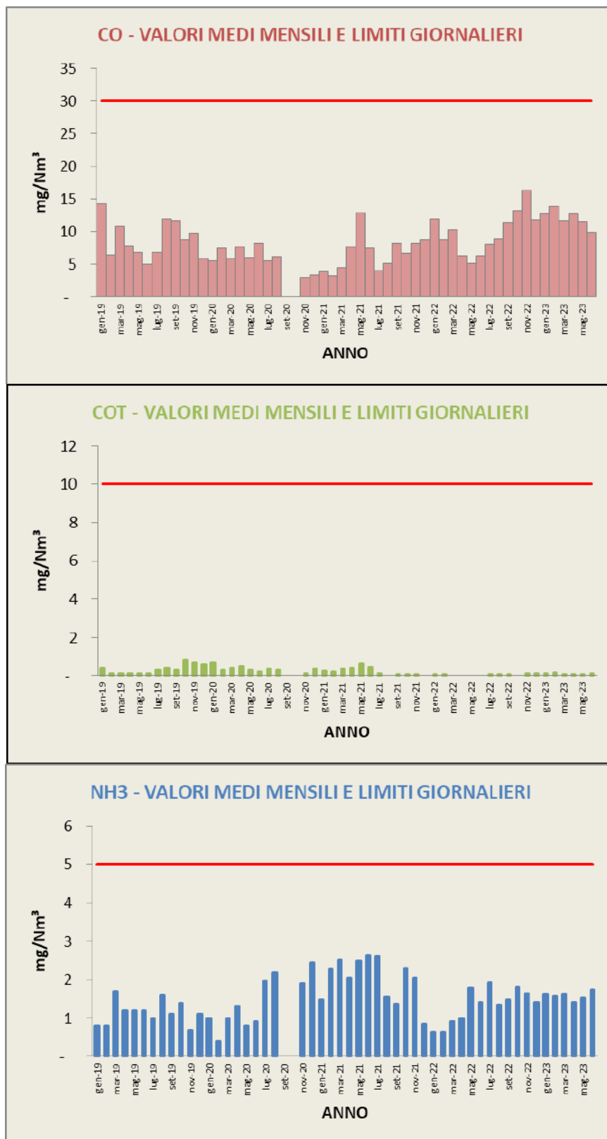
Grafici 27, 27a e 27b: Valori medi e limiti per impianto a pieno regime di CO, COT e NH 3
