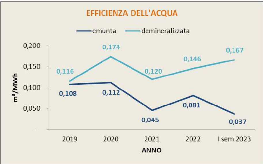
Grafico 16: Efficienza dell'acqua emunta e demi
