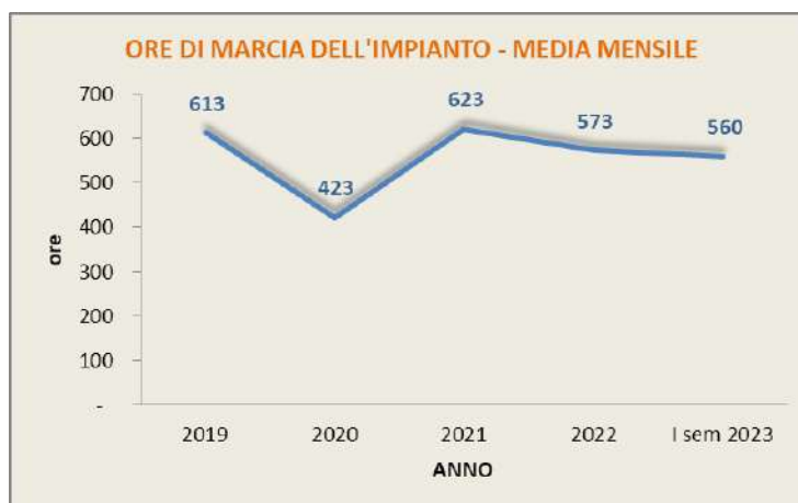
Grafico 6: Ore di marcia dell'impianto - media mensile
