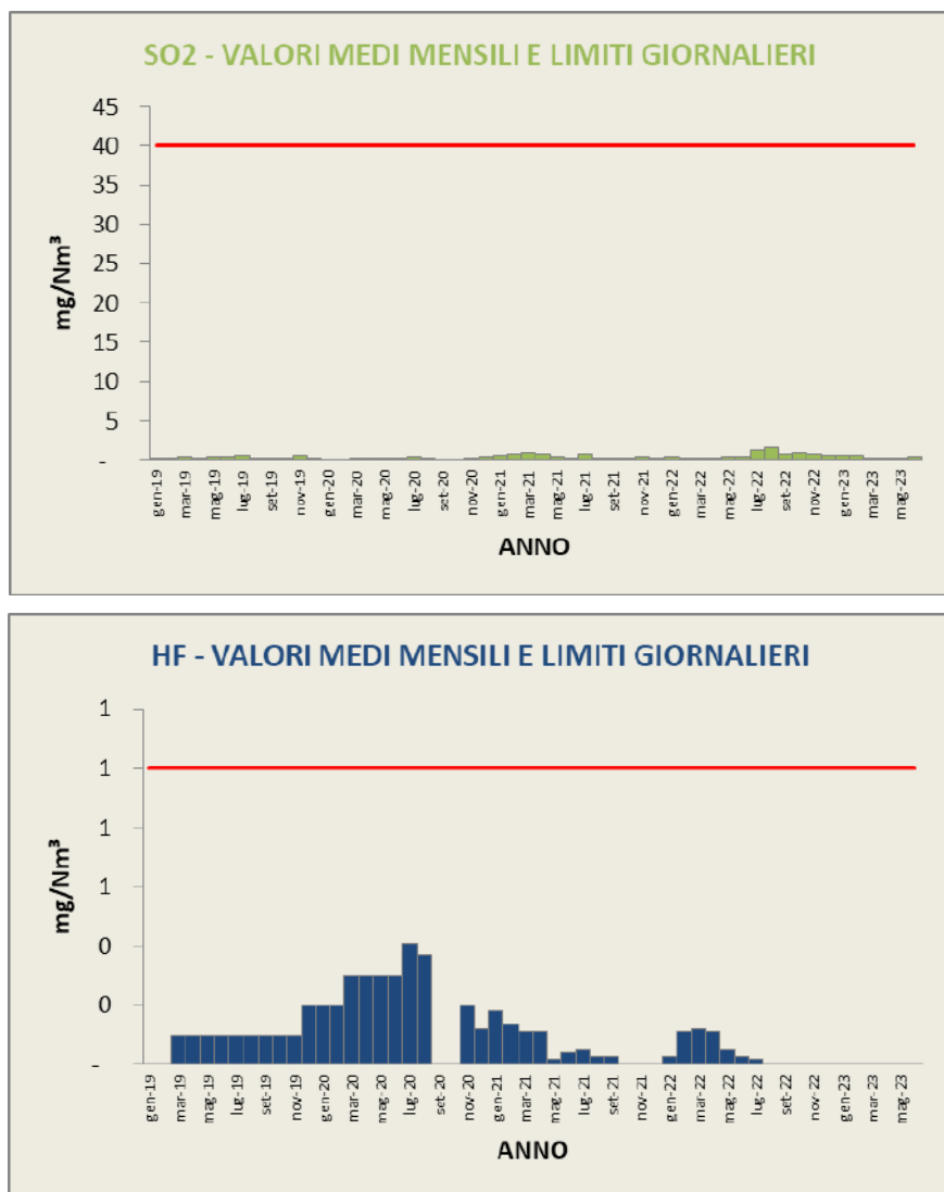
Grafici 30 e 30a: Valori medi e limiti per impianto a pieno regime di SO2 e HF
