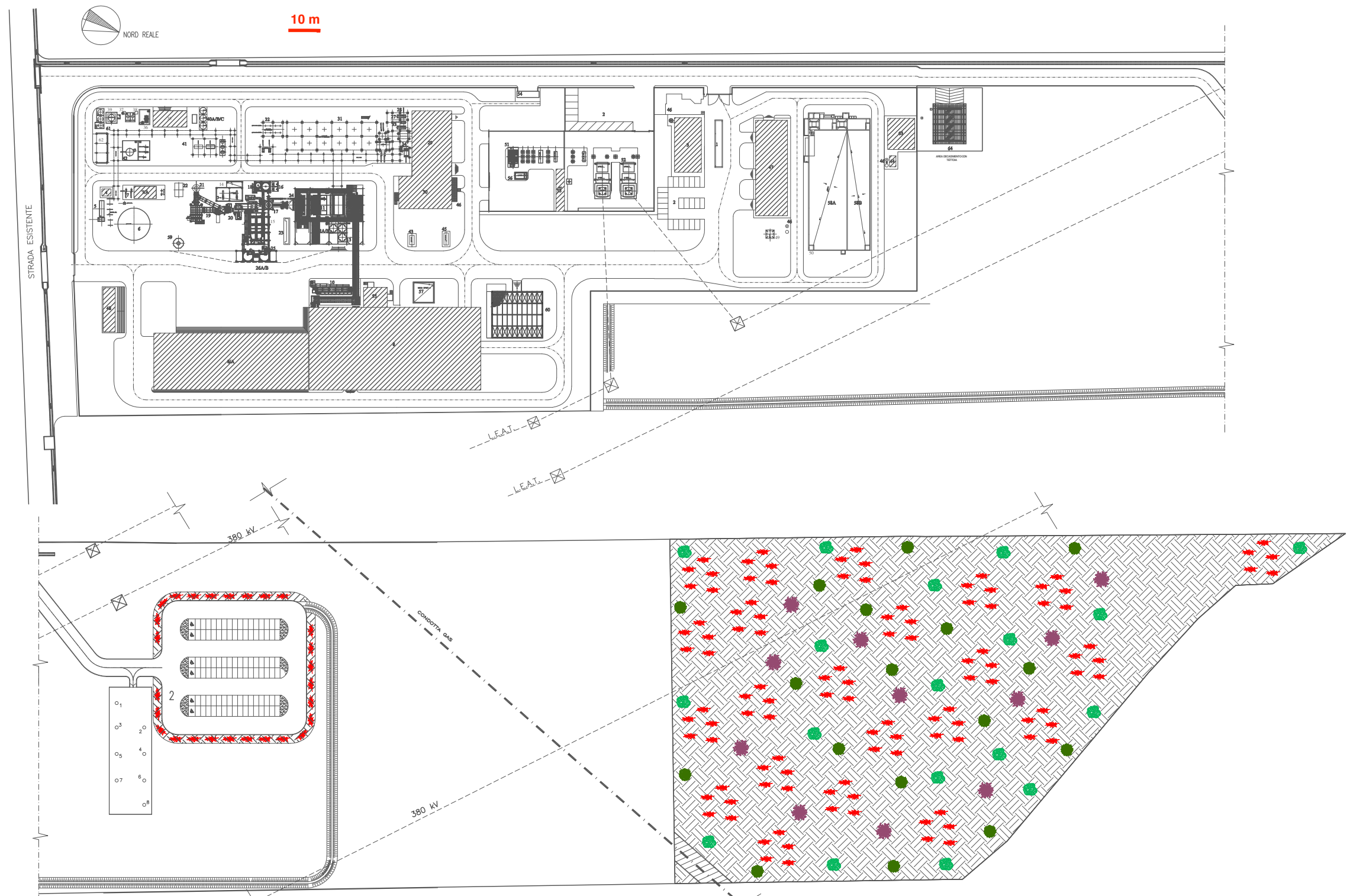
Fig. n. 3 - Planimetria Impianto di Produzione di Energia Elettrica – E.T.A. S.r.l.
