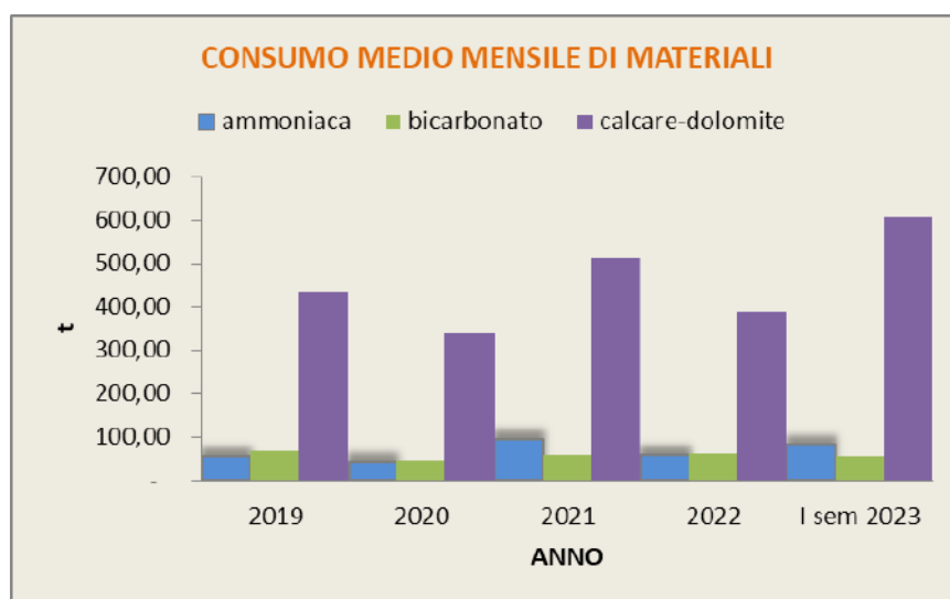
Grafico 10: Consumo ammoniaca, bicarbonato e calcare dolomite
